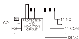
接线图 / Wiring diagrams
