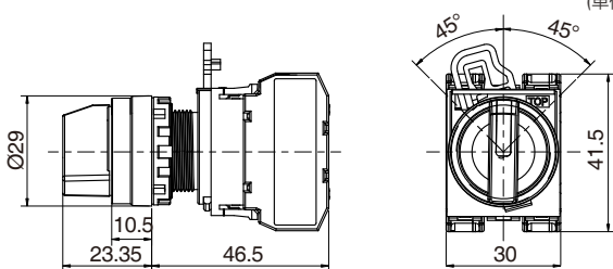
3P选择开关 3P Selector Switches
