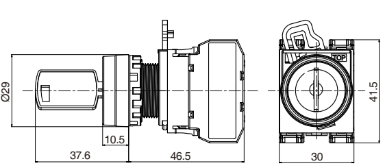
3P钥匙开关 3P Key Switches
