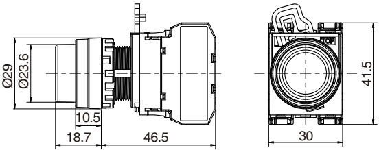
高头按钮 Flush Pushbuttons
