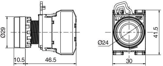
平头按钮 Flush Pushbuttons
